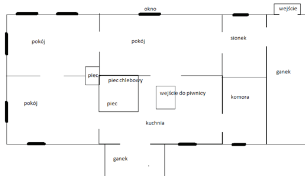
Rys. 2. Plan chałupy dwutraktowej, symetrycznej z gankiem (nr. 92), rys. Gintare Dąbrowska
