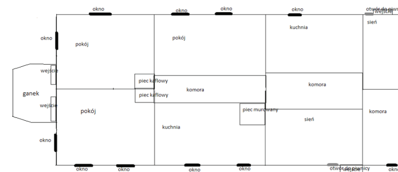
Rys. 7. Plan dom murowanego, o konstrukcji szkieletowej, dwutraktowy, asymetryczny, rys. Gintare Dąbrowska
