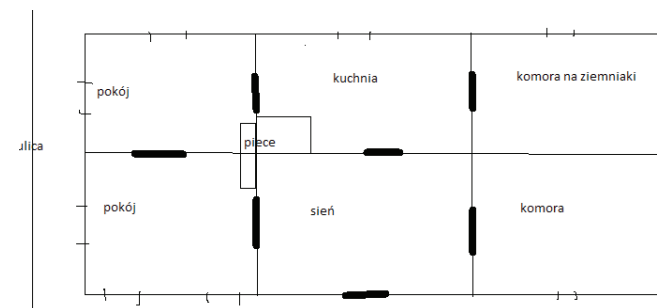
Rys. 5. Plan chałupy dwutraktowej, symetrycznej (nr. 207), rys. Gintare Dąbrowska
