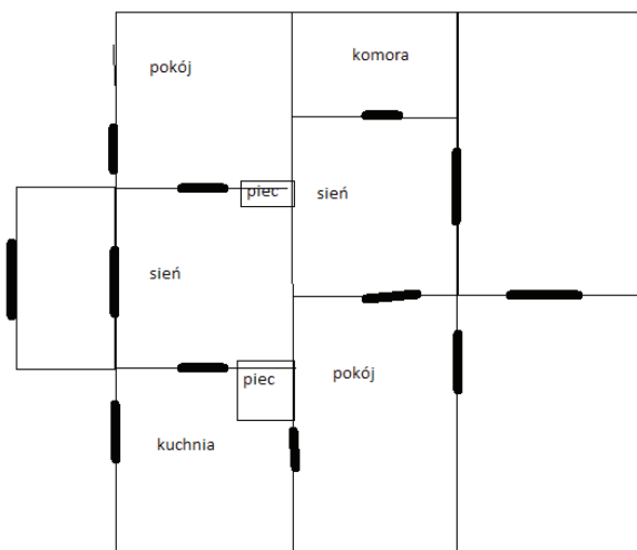
Rys. 3. Plan chałupy dwutraktowej symetrycznej (nr. 176), rys. Gintare Dąbrowska
